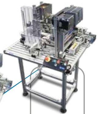
HAS-204 SE I4.0
